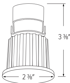
E1L61 - 1" ROUND TRIMLESS
